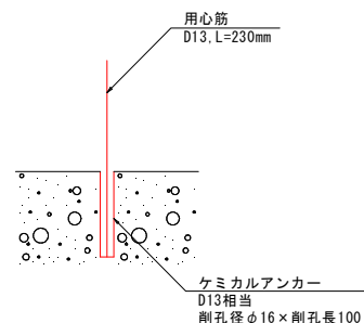
差し筋詳細図 S=1:5
